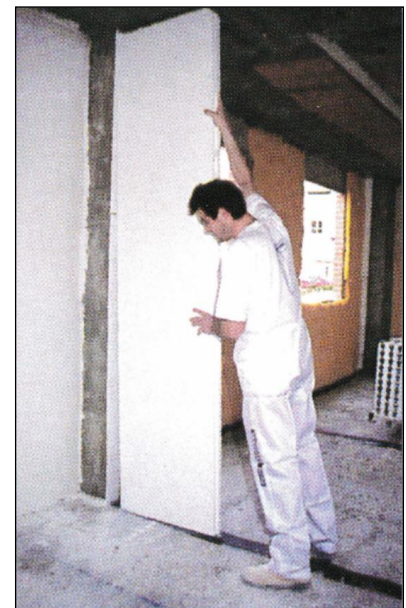
Fig. 3: Proceso de puesta en obra de un panel enterizo de escayola
