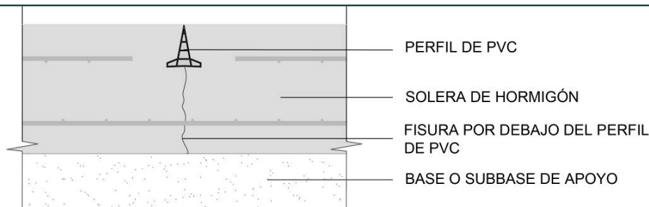
Figura 14. Detalle junta de retracción con perfil de PVC
