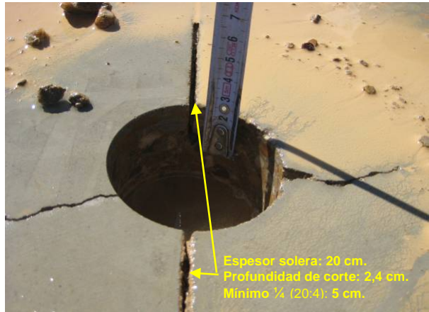
Figura 6. Fisuración de retracción, deficiente profundidad de corte
