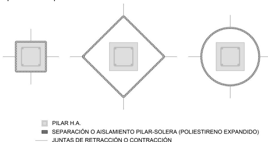
Figura 12. Detalle juntas de separación o aislamiento entre la solera y otros elementos constructivos
