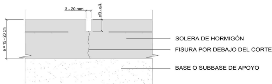
Figura 13. Detalle junta de retracción por serrado del hormigón
