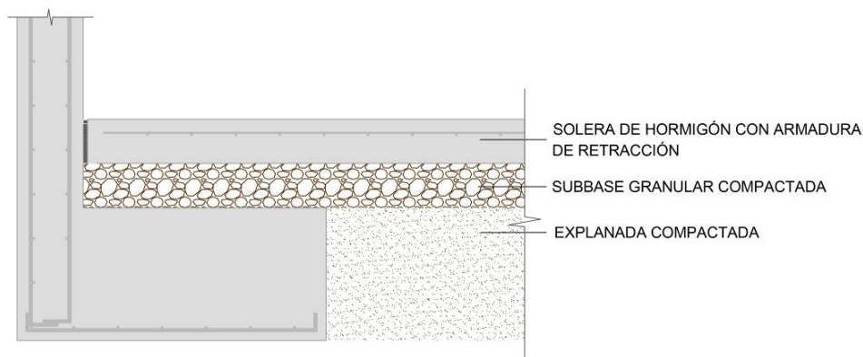
Figura 11. Detalle encuentro solera con elementos de cimentación (Zapatas)
