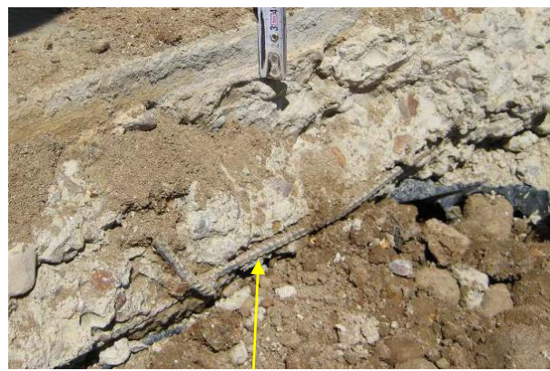
Figura 4: Incorrecta colocación del armado.
