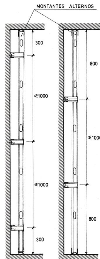
Fig. 7: Disposición al tresbolillo de las piezas de arriostramiento en un trasdosado autoportante. Ejemplo de acotación para una altura de 2,60m.
