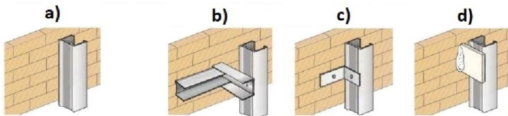
Fig. 5: Interrelación entre los montantes del trasdosado y el trasdós del muro-base. ▪ Montantes libres -no arriostrados- (a); ▪ Montantes arriostrados: con doblado de trozo de otro montante (b), con perfil angular (c), con lambeta o cartela (d).
